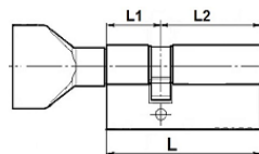
Обозначение несимметричных цилиндров - NW L1/L2
