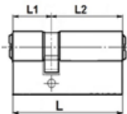
Обозначение несимметричных цилиндров - C L1/L2
