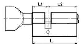
Обозначение несимметричных цилиндров - CW L1/L2
