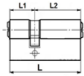
Обозначение несимметричных цилиндров - N L1/L2
